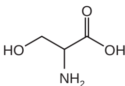
serine ( ser )
